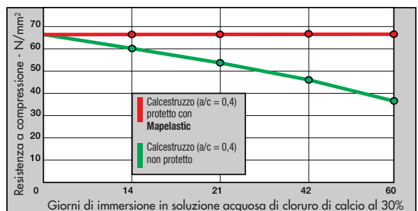
Fig. 4: Effetto di Mapelastic sul decadimento meccanico del calcestruzzo dovuto ai sali disgelanti a base di cloruro di calcio
