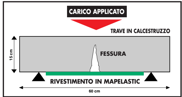
Fig. 1: Protezione con Mapelastic di una fessura all'intradosso di una trave in calcestruzzo sottoposta ad una sollecitazione flessionale
