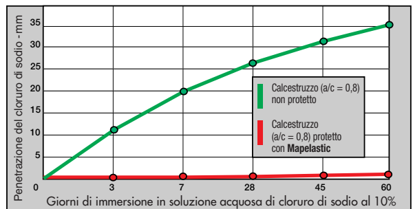
Fig. 3: Effetto di Mapelastic sulla penetrazione del cloruro di sodio in un calcestruzzo poroso
